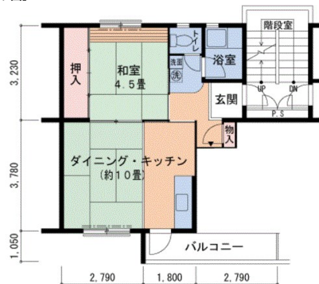
【間取り図】
