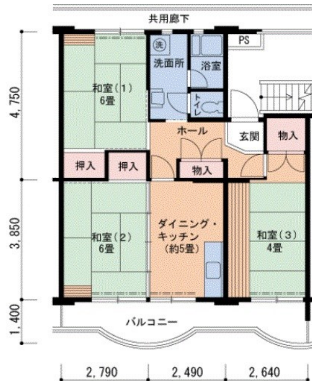
【間取り図】
