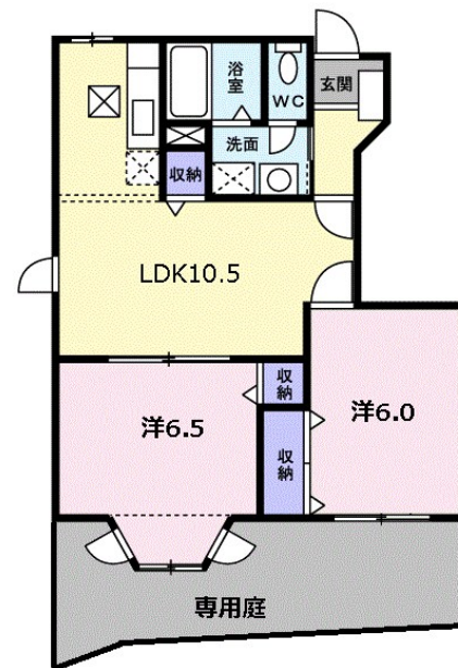
【間取り図】
