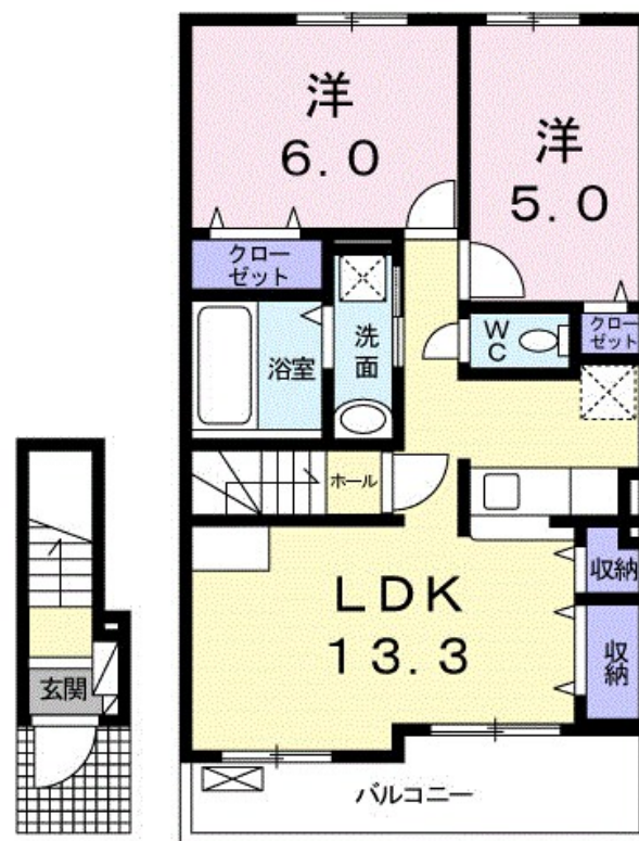
【間取り図】
